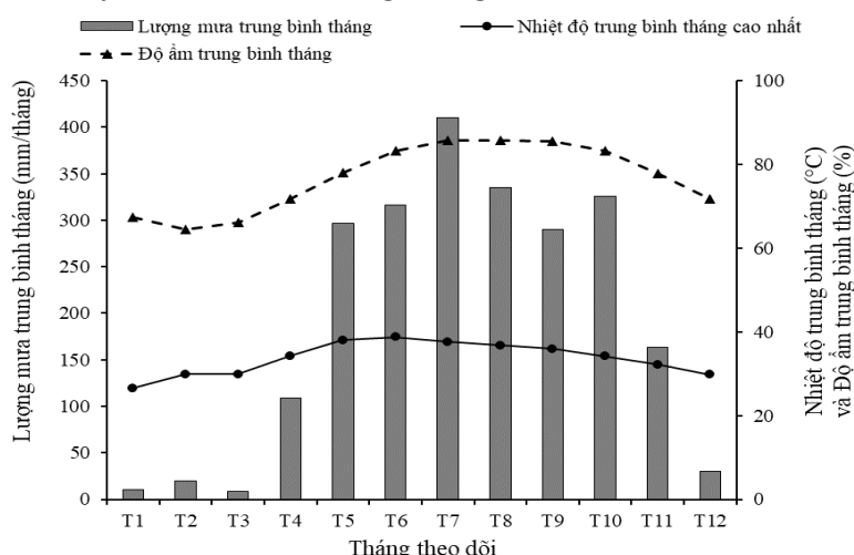
Hình 1. Lượng mưa trung bình tháng, nhiệt độ trung bình tháng và độ ẩm trung bình tháng trong 5 năm (2013-2017) tại trạm Khí tượng Thủy văn Đồng Xoài
